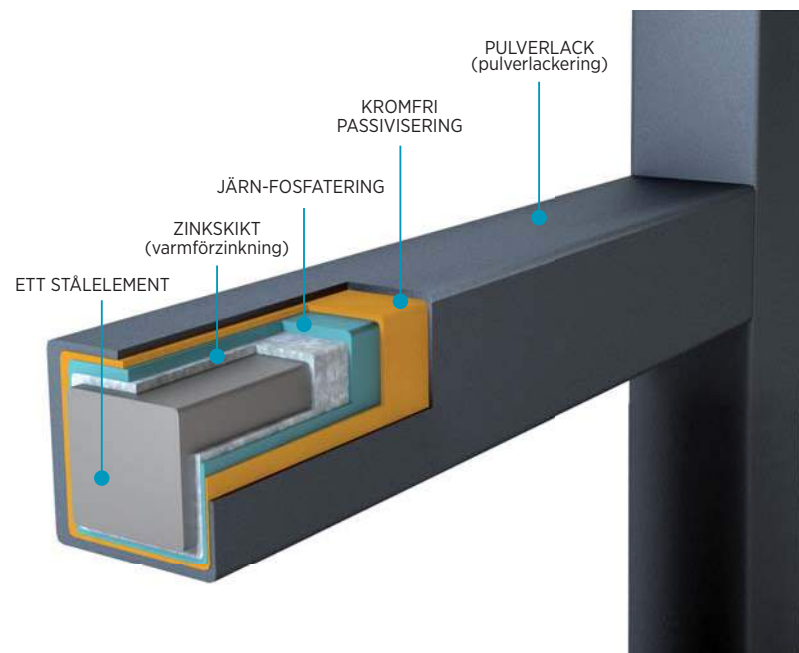
Sektion genom ett elementet säkrat i DUPLEX-system
